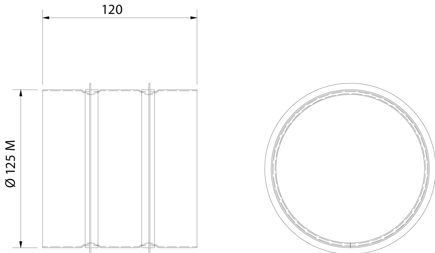
ALVEOLAR 125mm spojka rozměry
