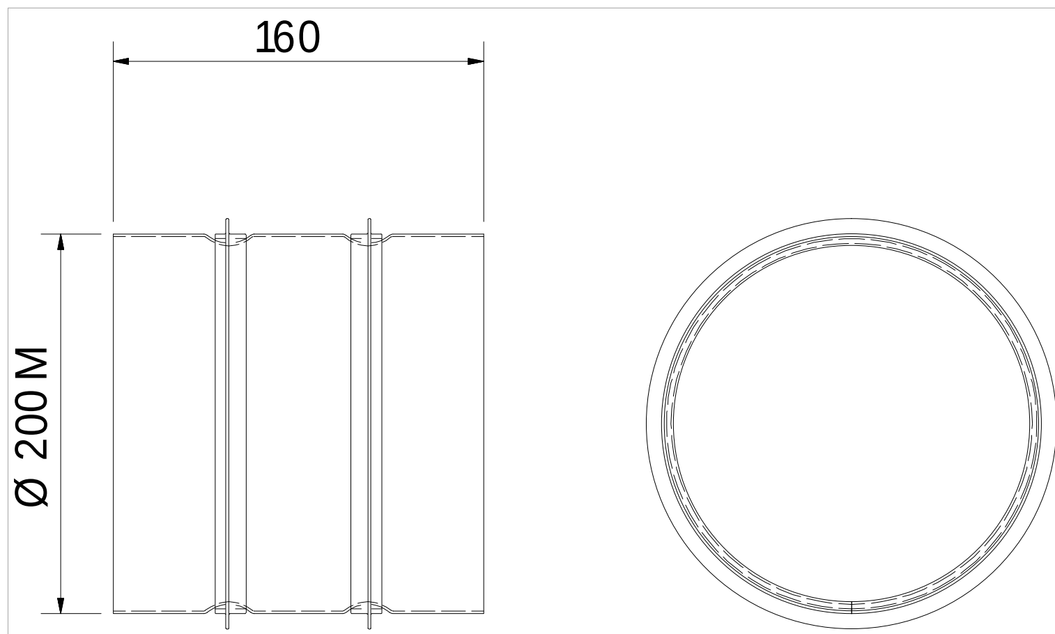
ALVEOLAR 200mm spojka rozměry
