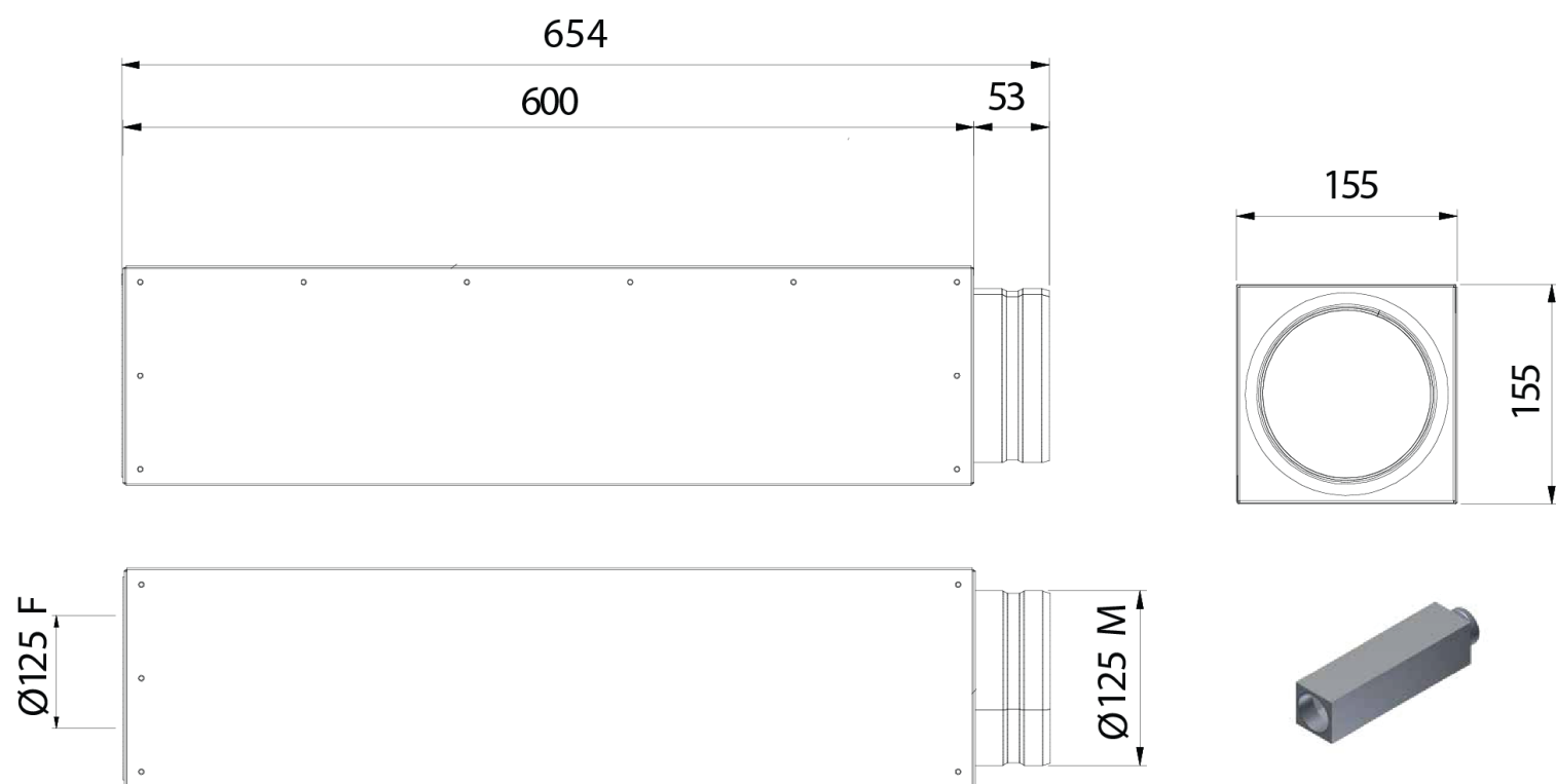
ALVEOLAR 125x600 tlumič rozměry
