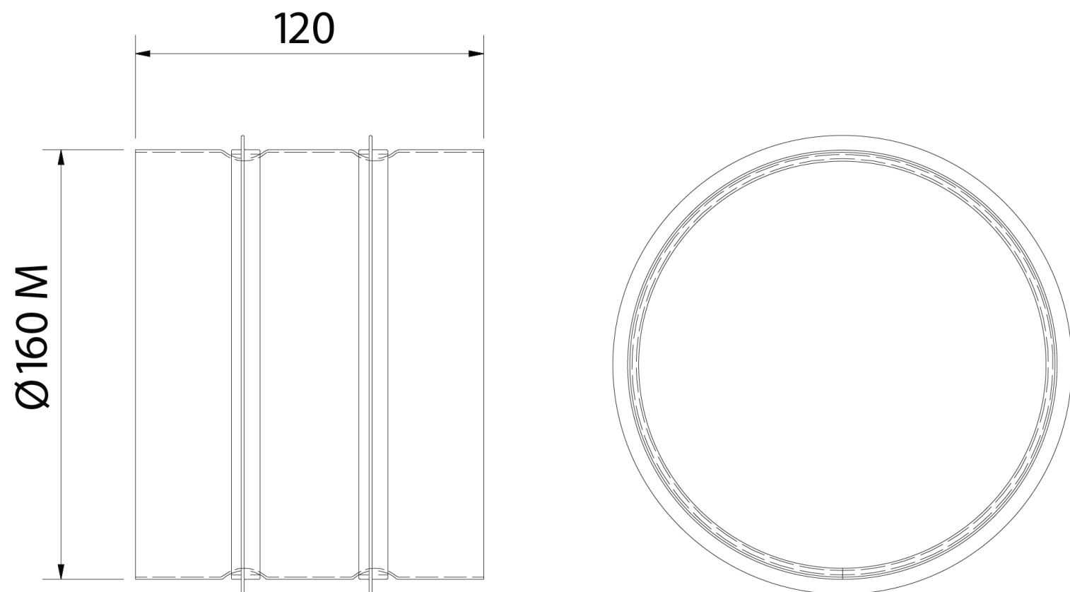
ALVEOLAR 160mm spojka rozměry
