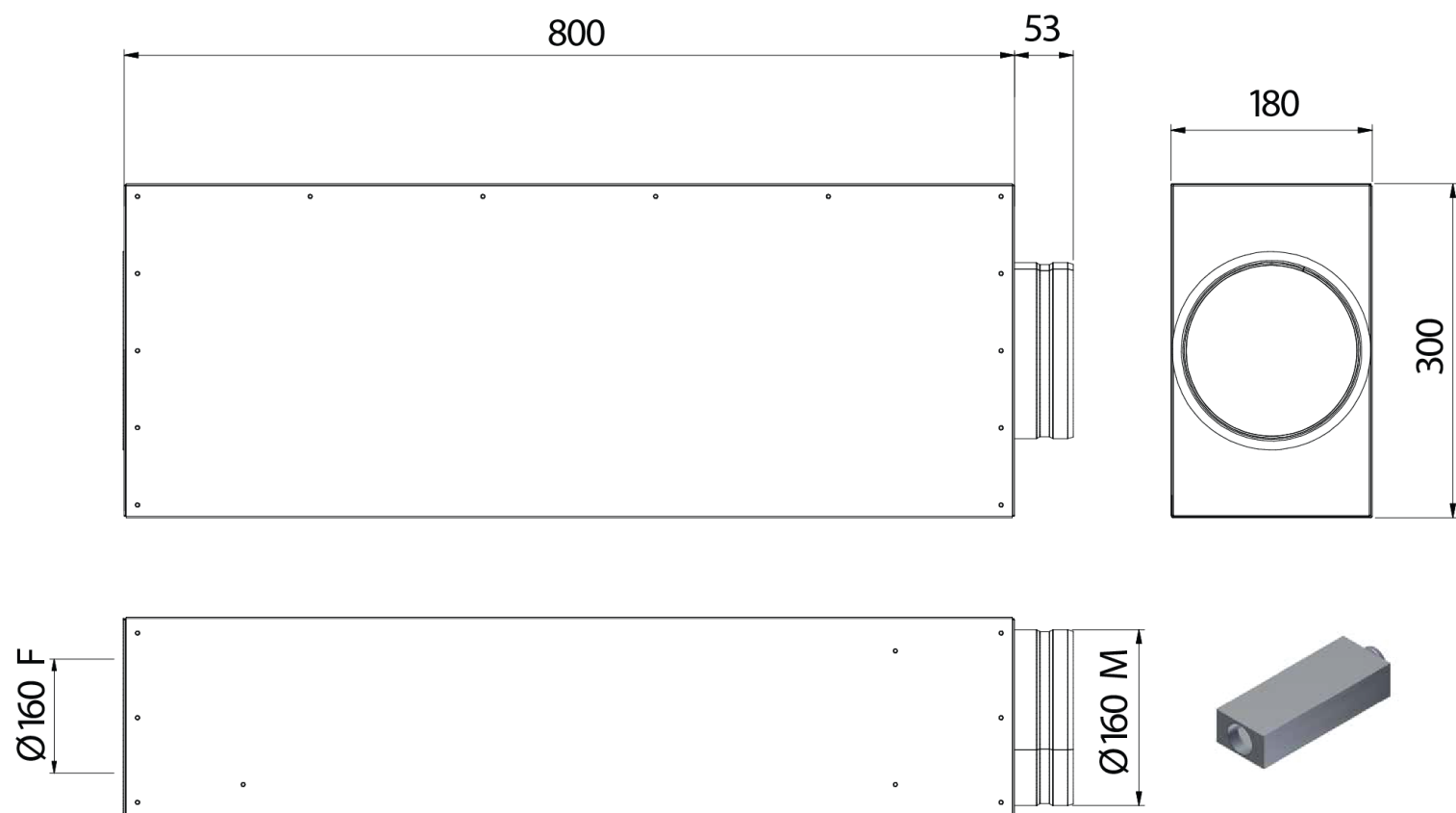
ALVEOLAR 160x800 tlumič rozměry
