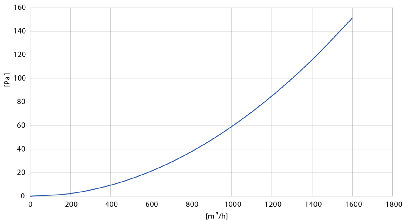
ALVEOLAR 160x800 tlumič tlakové ztráty
