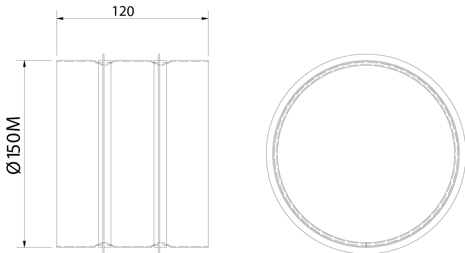
ALVEOLAR 150mm spojka rozměry
