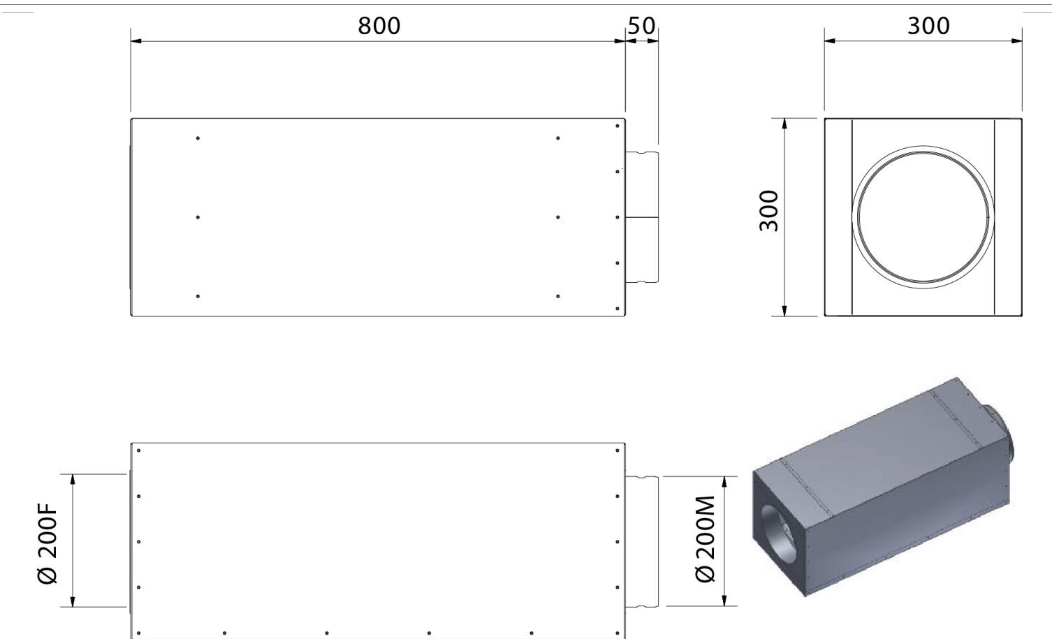
ALVEOLAR 200x800 tlumič rozměry
