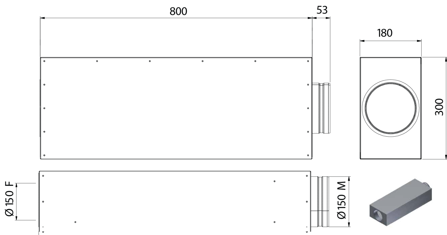
ALVEOLAR 150x800 tlumič rozměry
