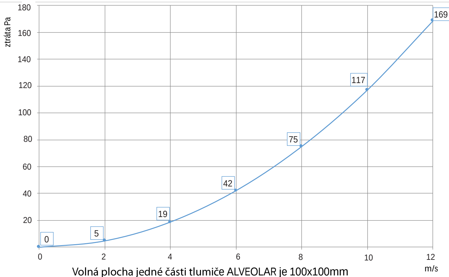
ALVEOLAR tlakové ztráty
