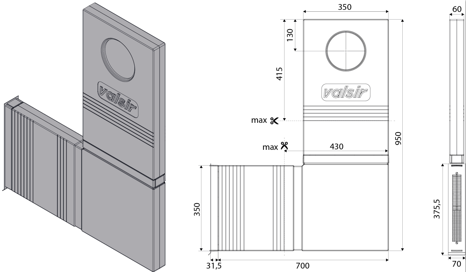
ANGOLARE rozměry
