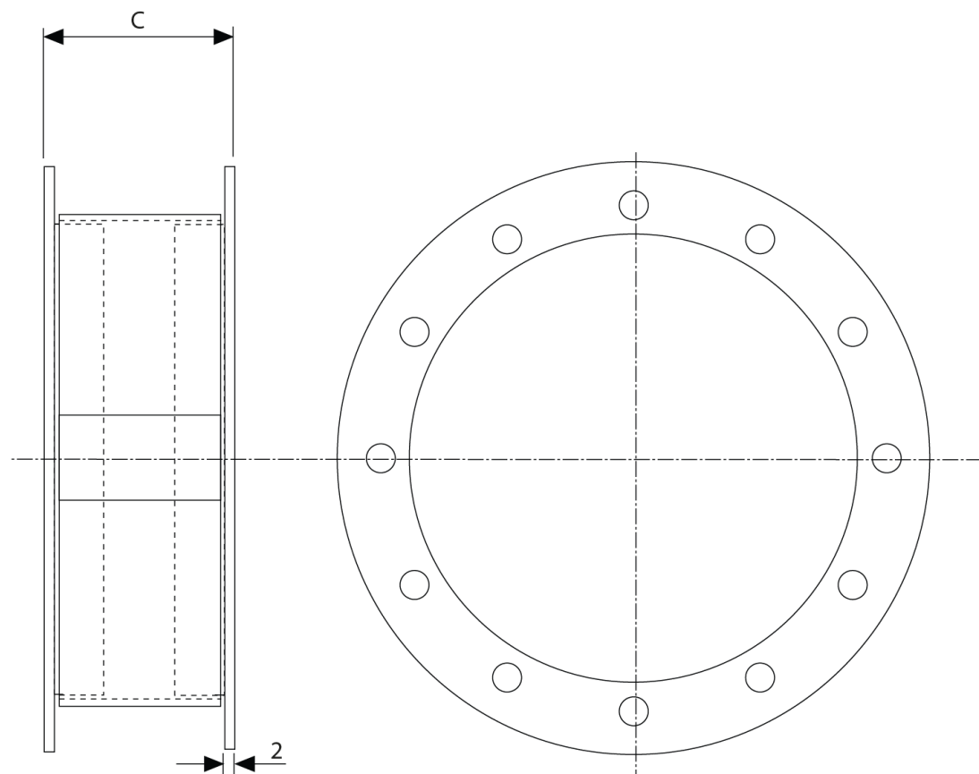
JM/JMv serie manžeta rozměry
