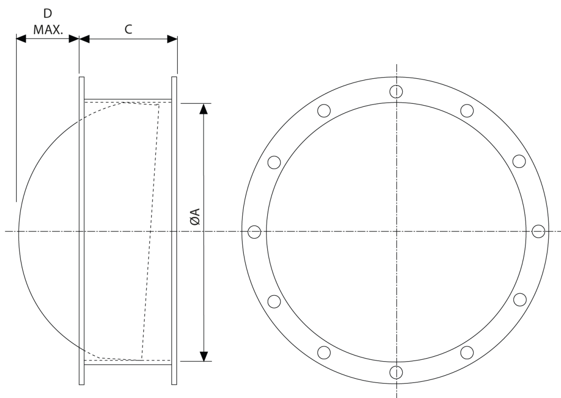
JM/JMv klapka rozměry
