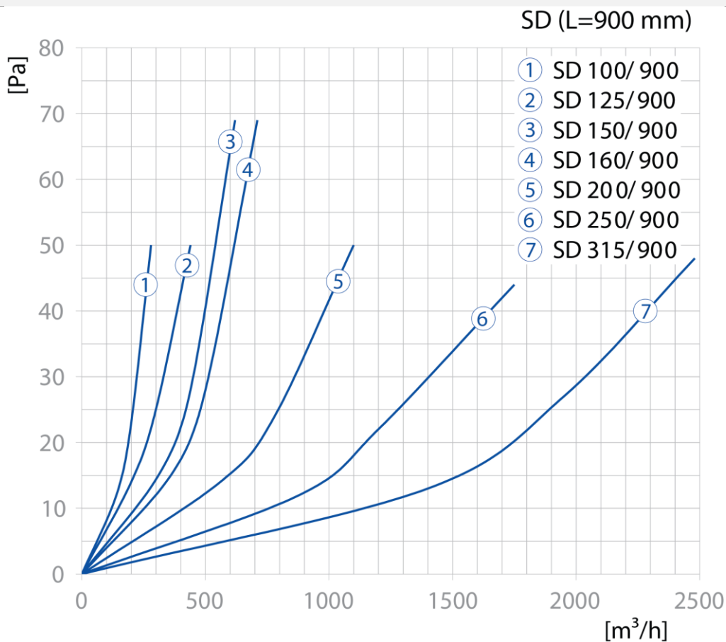
SD kruhové 900mm ztráta tlaku
