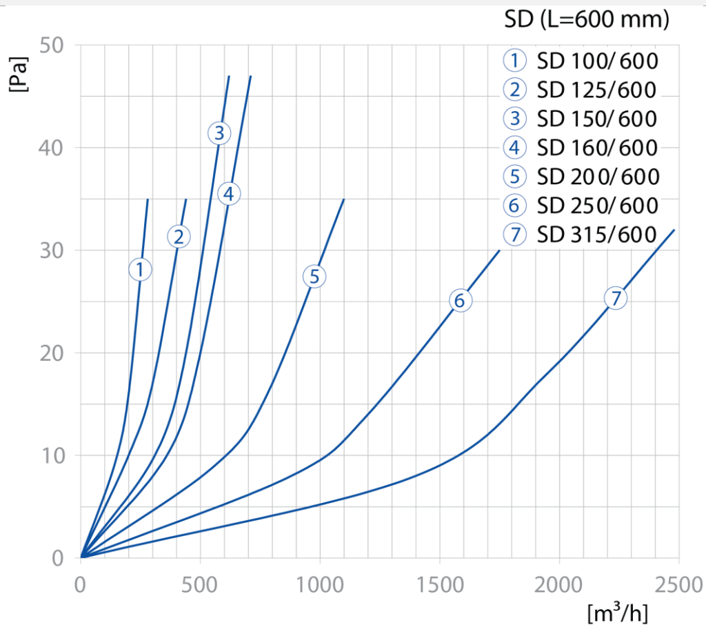
SD kruhové 600mm ztráta tlaku
