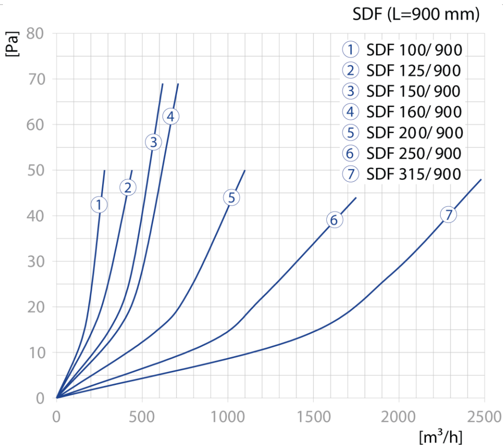
SDF délka 900mm ztráta tlaku
