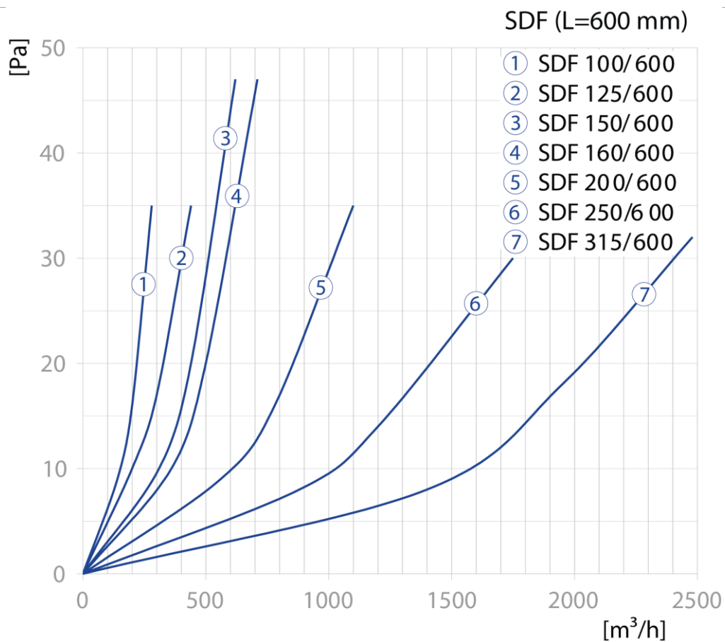
SDF délka 600mm ztráta tlaku
