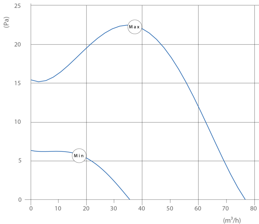
Silent Fan výkon
