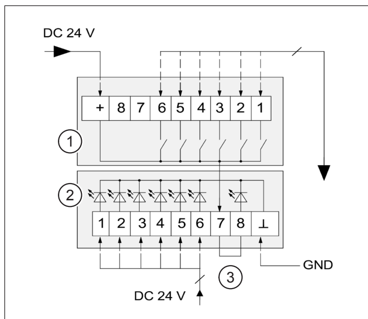
Obr. 4: Schéma zapojení dotykového senzoru InControl
