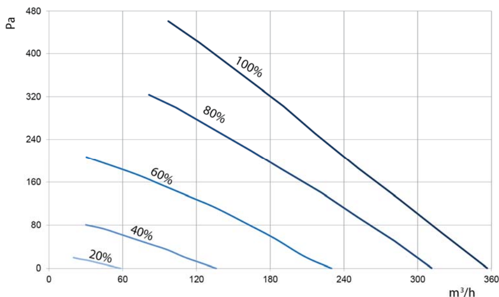
Obr.6.d Křivka příjmu dle reg.č. 1253/2014 (ErP).
