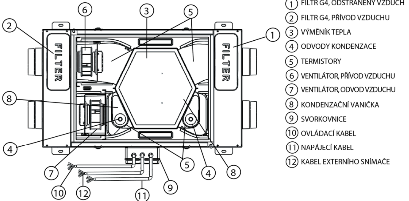
Obr. 8.a Vnitřní součásti
