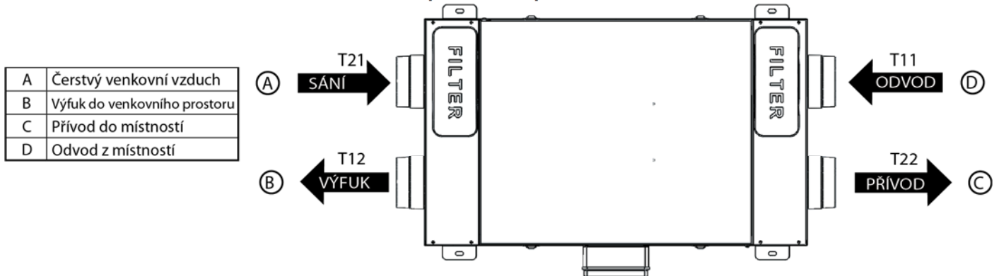
Obr. 7.a Teplotní sondy
