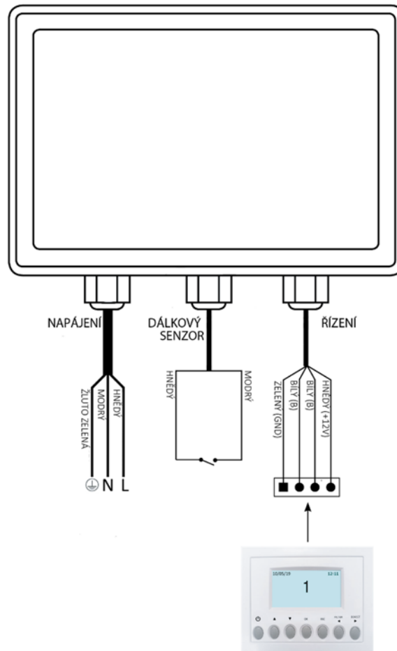
Obr. 5.f Elektrické připojky
