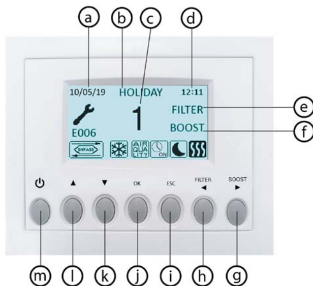
Obr. 7.c CTRL-DSP
