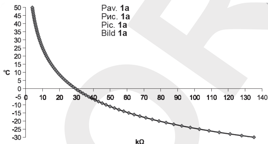
Obrázek 1a : Závislost mezi odporem snímače teploty a naměřenou teplotou vzduchu Typ snímače : NTC 10 K 10 kΩ při 25 °C; \beta = 3380 \text{ K}
